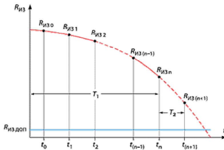
Сопротивление изоляции в зависимости от времени Рис. 3
