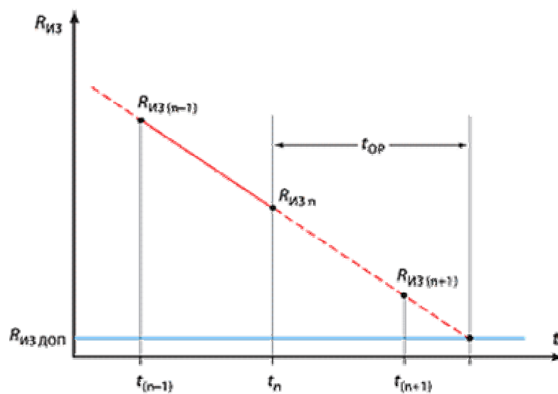
Графическая интерпретация аналитического прогнозирования сопротивления изоляции Рис. 4
